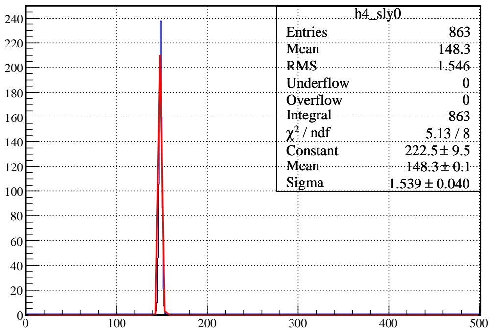
図 2 Gaussian で pedestal のフィット
