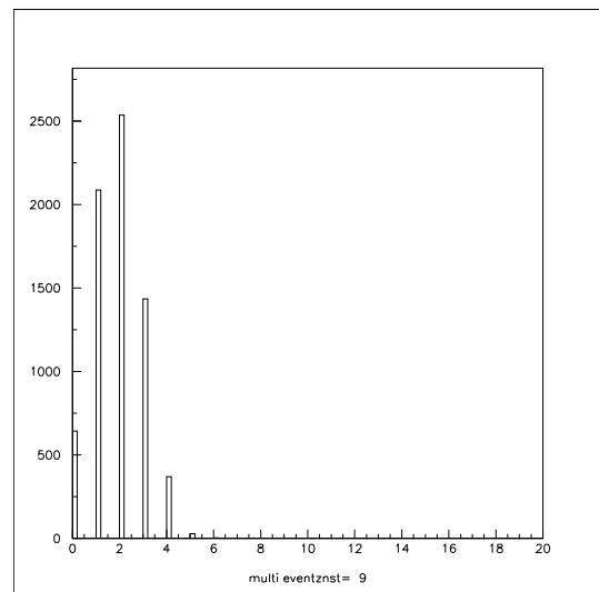
図 0.8 neutron counter が 8 つ (thr6.0MeV)
